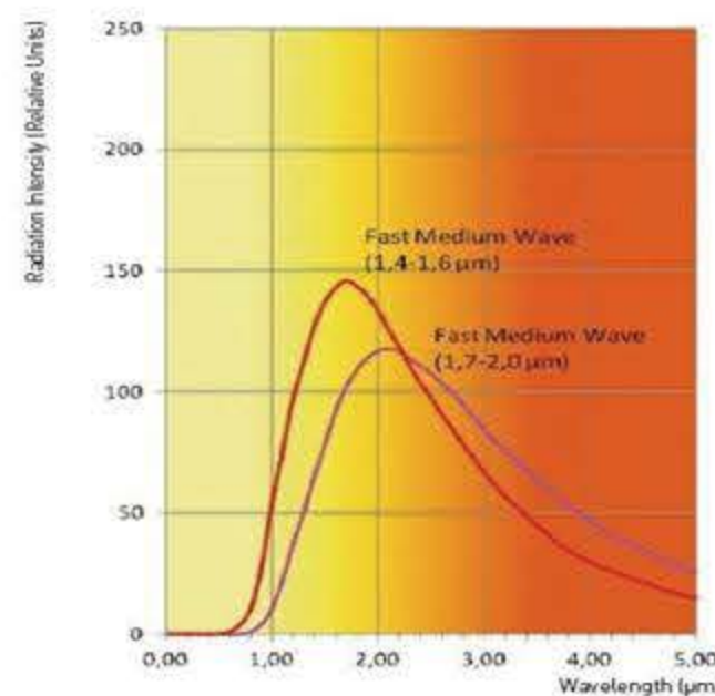
红外快中波石英管
